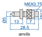
anvils
